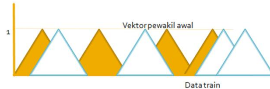
Gambar 6. Fuzzy intersection dari vektor referensi FLVQ dengan vektor masukan.
