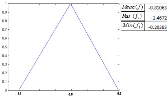
Gambar 4. Vektor Fuzzy .
