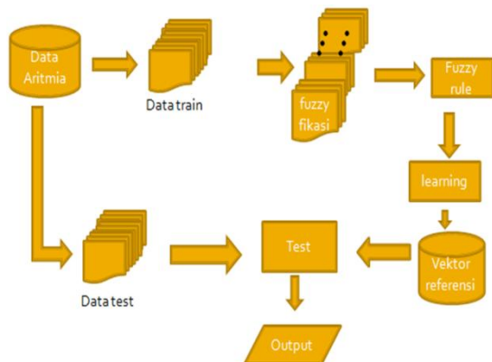
Gambar 9. Blok diagram sistem klasifikasi beat aritmia dengan FWLVQ.
