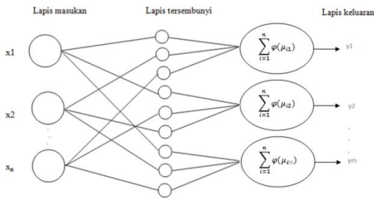
Gambar 8. Arsitektur FWLVQ.
