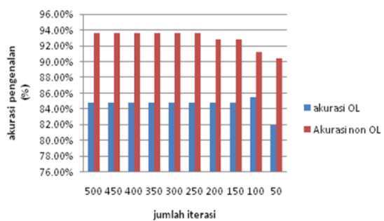
Grafik Akurasi (FLVQ)Pengenalan Beat Aritmia
